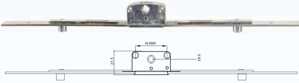
Casement Espag Rod Backset : 19.5mm Length : 400mm - 1800mm
